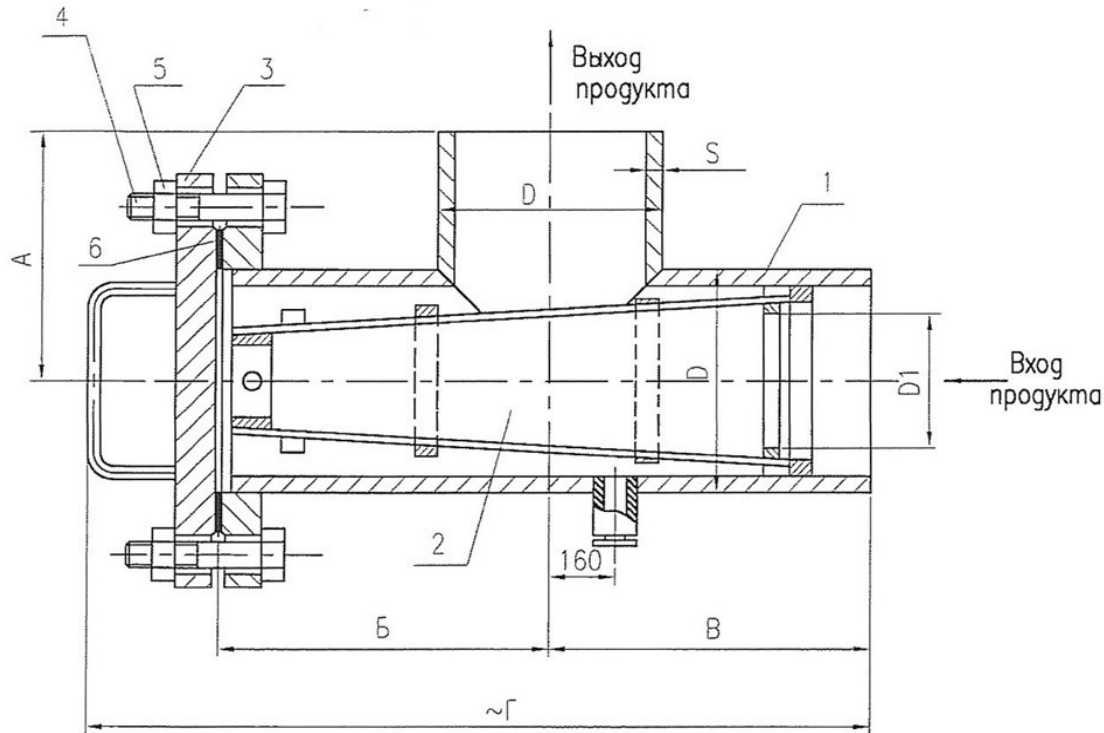
Рис. 5. Фильтр сетчатый типа V.
