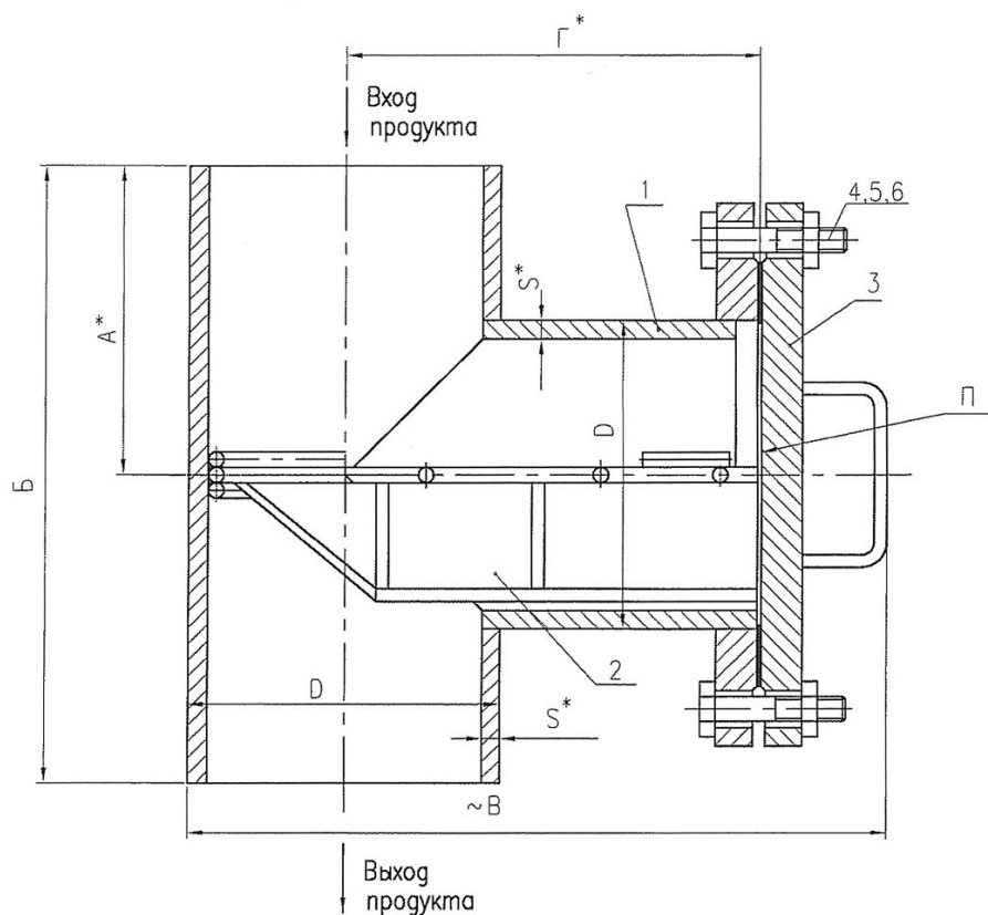
Рис. 4. Фильтр сетчатый типа IV.
