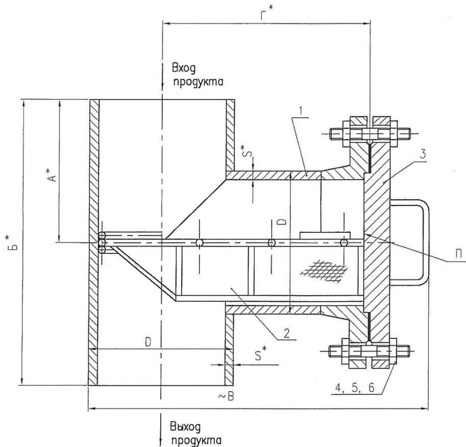
Рис. 1. Фильтр сетчатый типа I.
