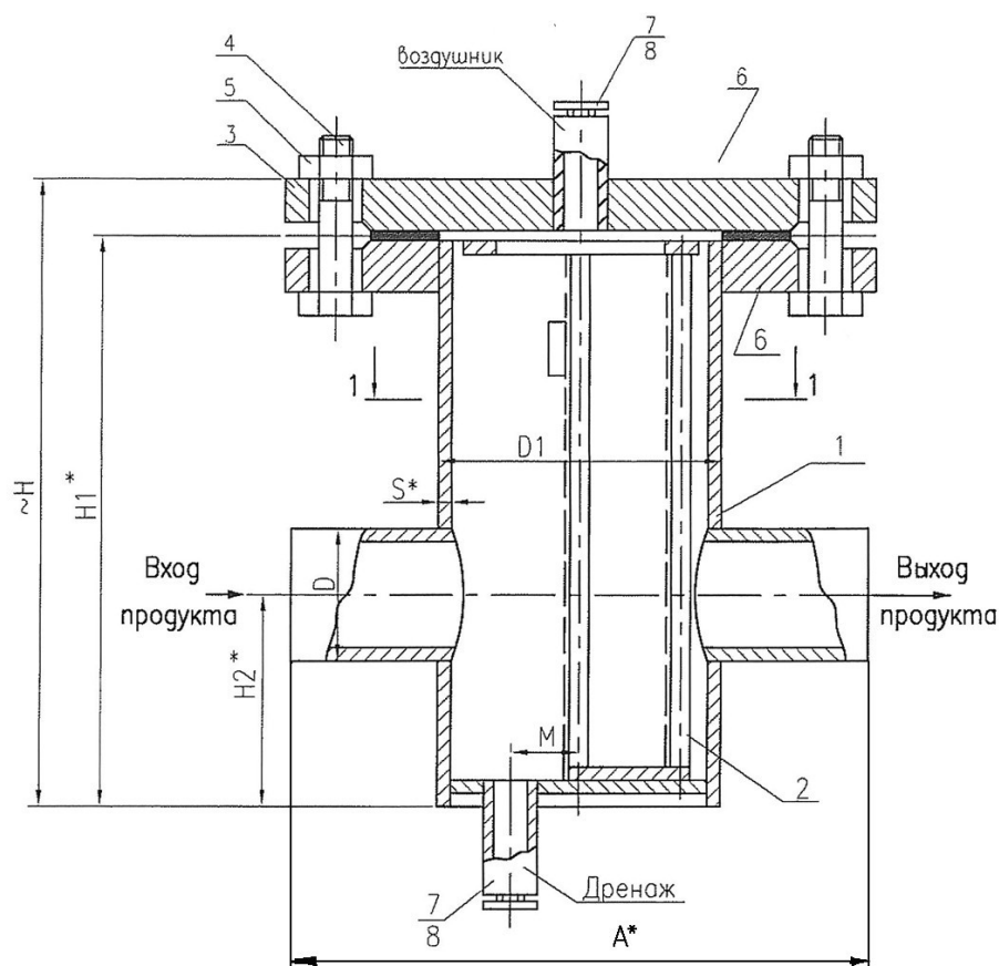
Рис. 6. Фильтр сетчатый типа VI.
