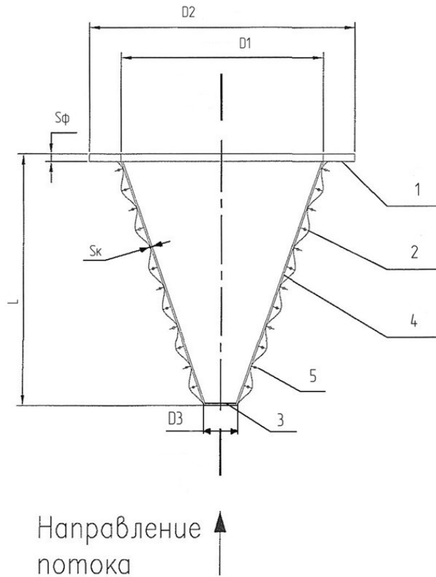
Рис. 7. Фильтр сетчатый временный тип В.
